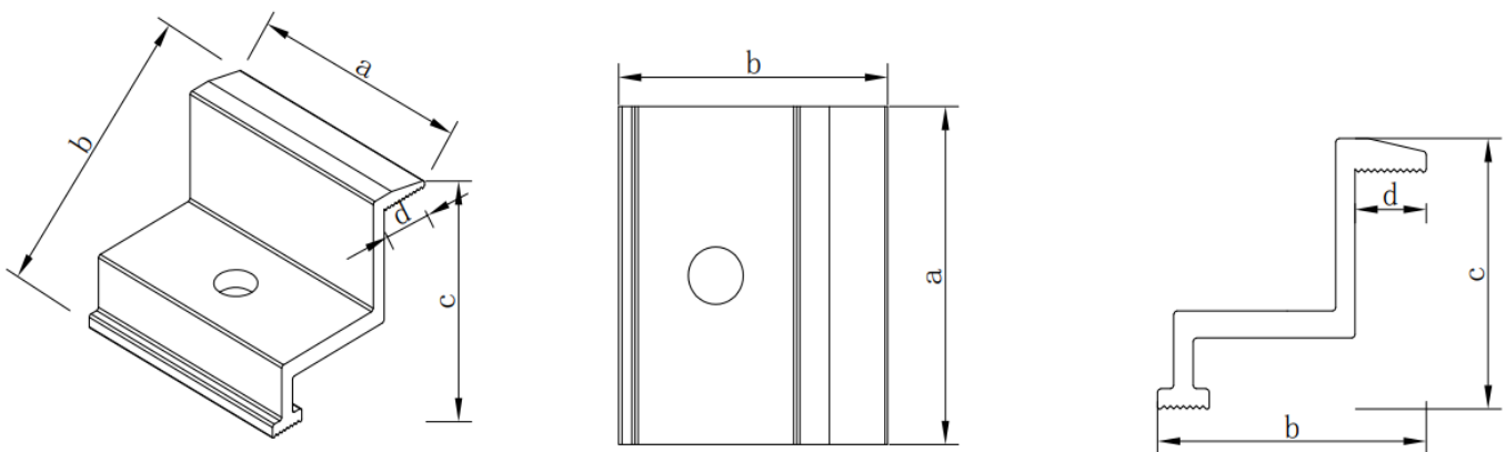
Fig. 5 Clamp
